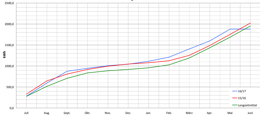
Solaretrag monatlich
